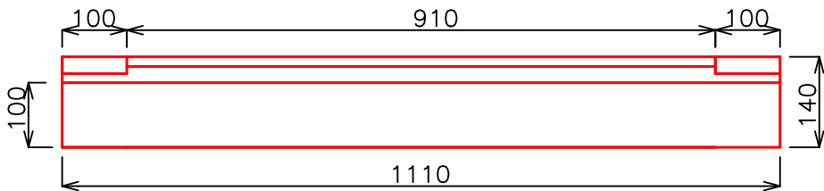
C3- CILL ELEVATION
