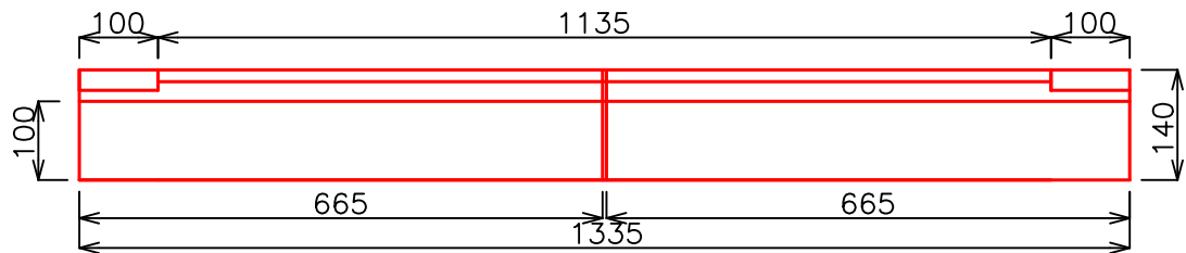
C2- CILL ELEVATION
