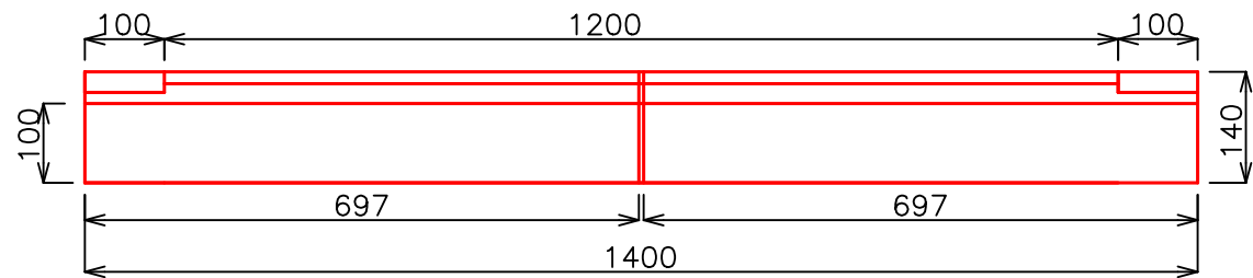
C1- CILL ELEVATION
