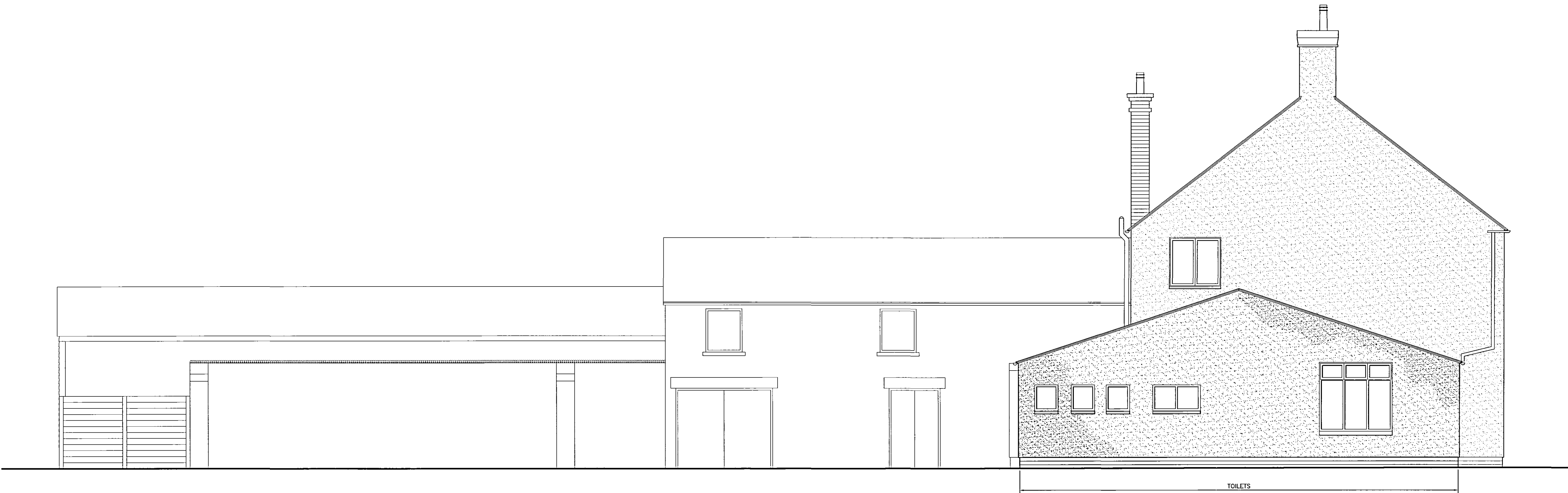
ELEVATION 'A'.
