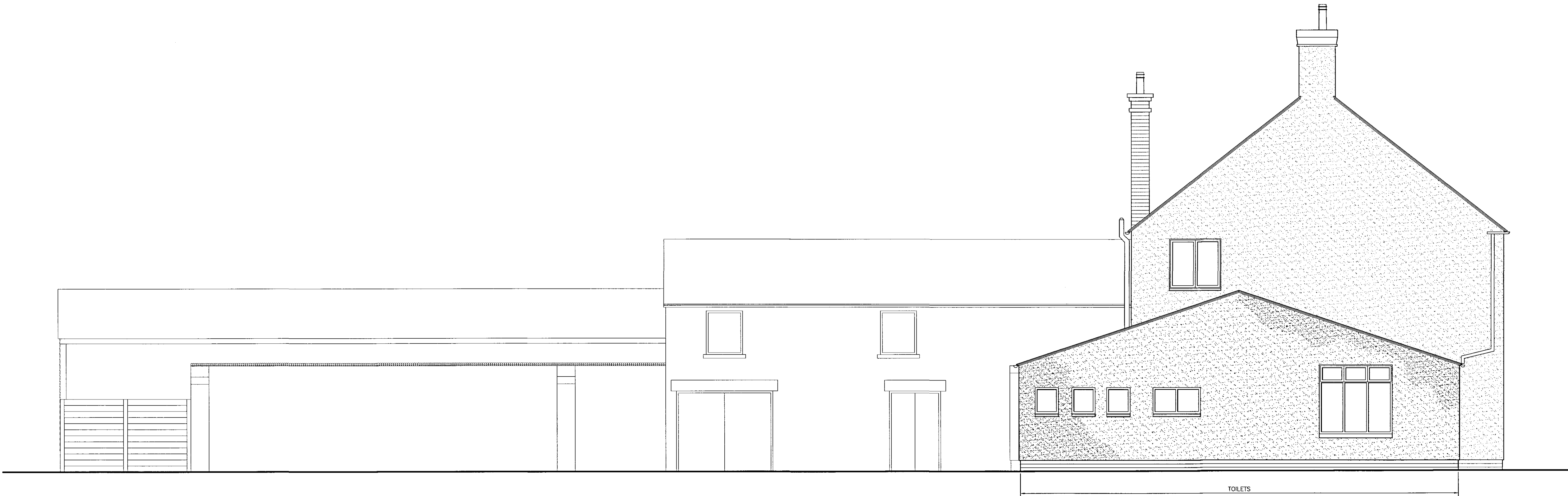
ELEVATION 'A'.
