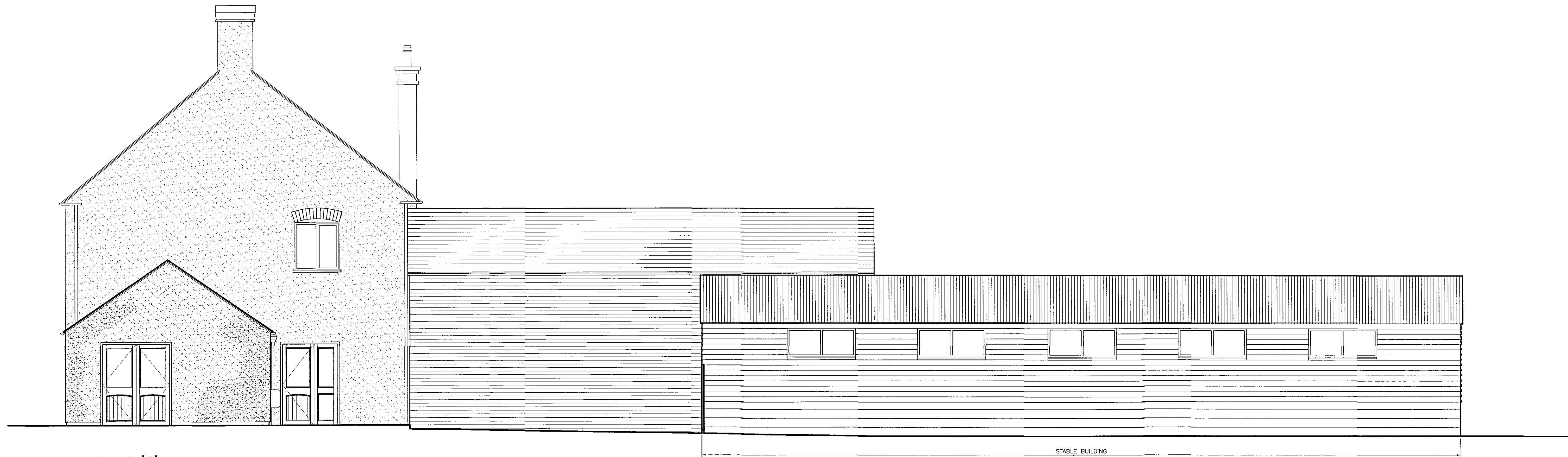
ELEVATION 'C'.
