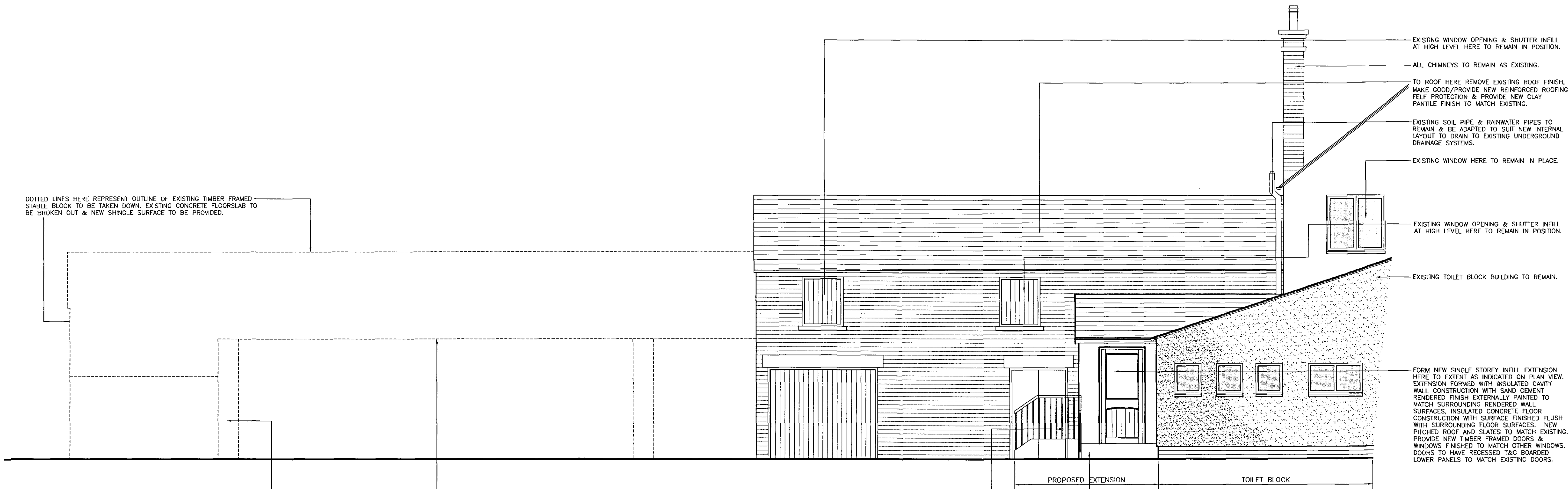
ELEVATION 'B'.
