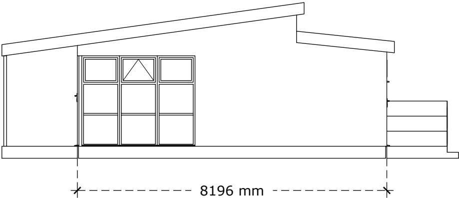
Right (N) elevation
