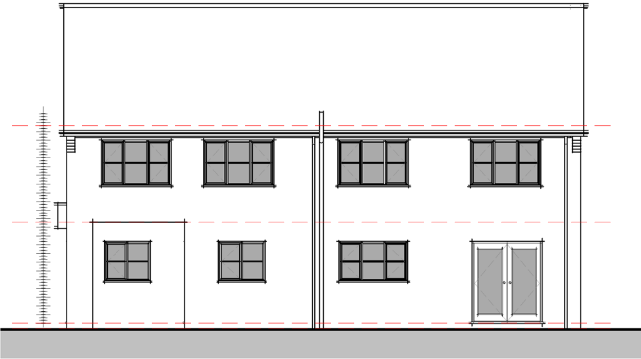
03 - Rear 1 : 100
