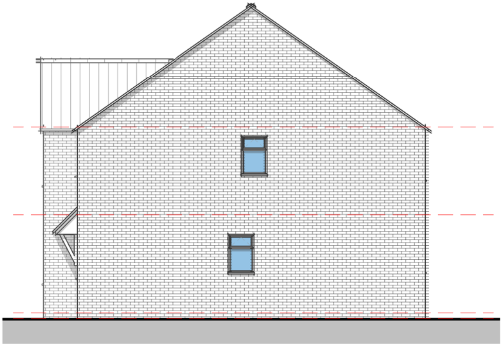
Elevation 02 - Right 1 : 100
