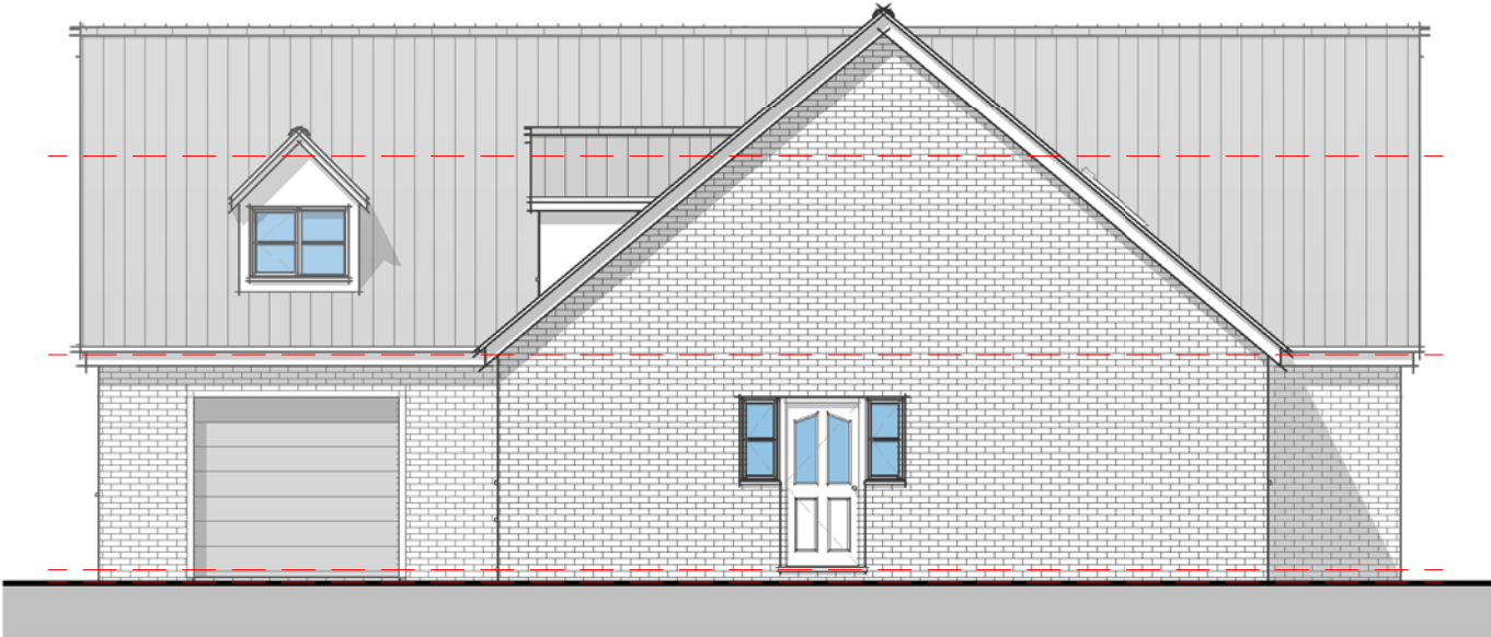
Elevation 02 - Right 1 : 100
