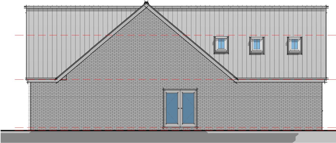
Elevation 04 - Left 1 : 100
